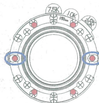
7.5Kフランジの場合
